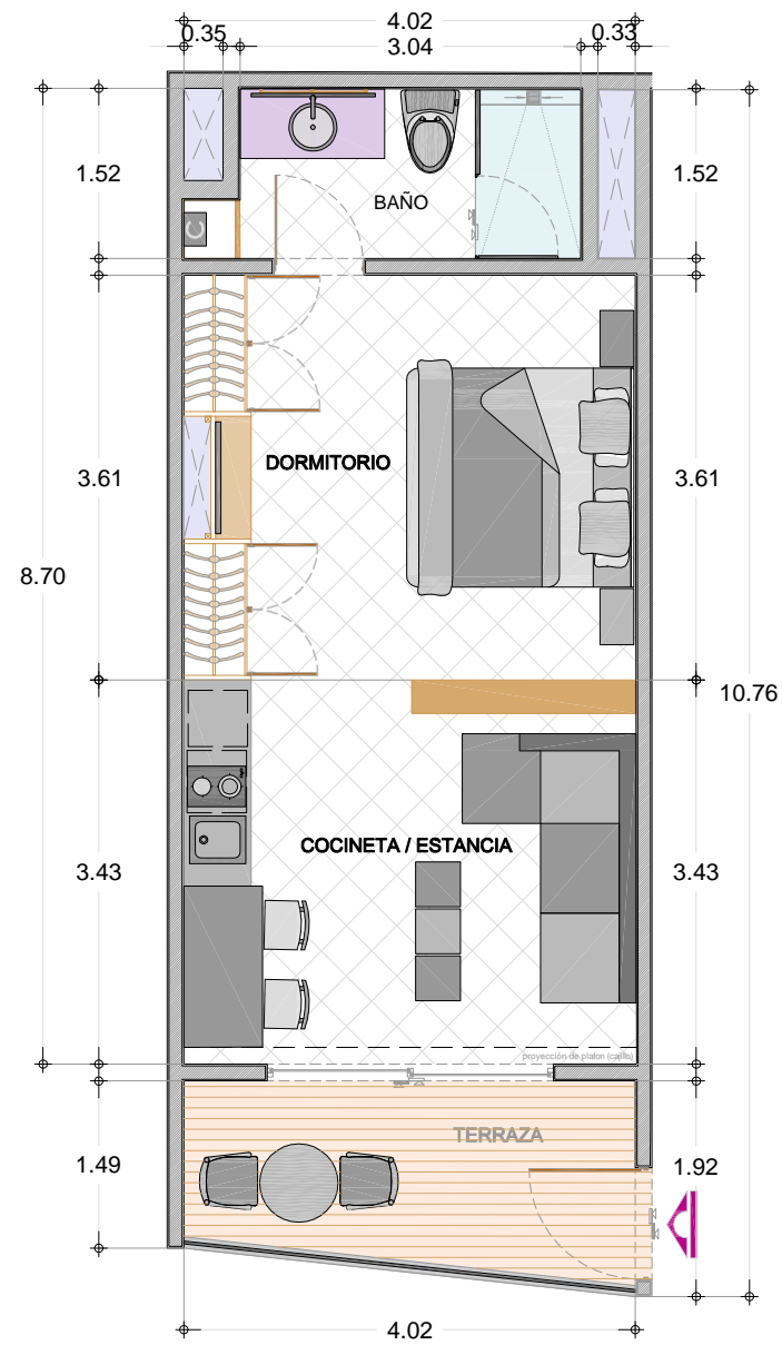
Planta TIPO 1
