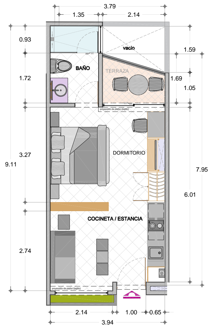
Planta TIPO 2A
