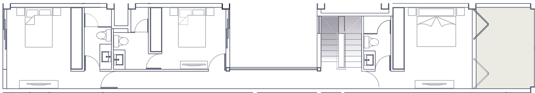
PLANTA ALTA
